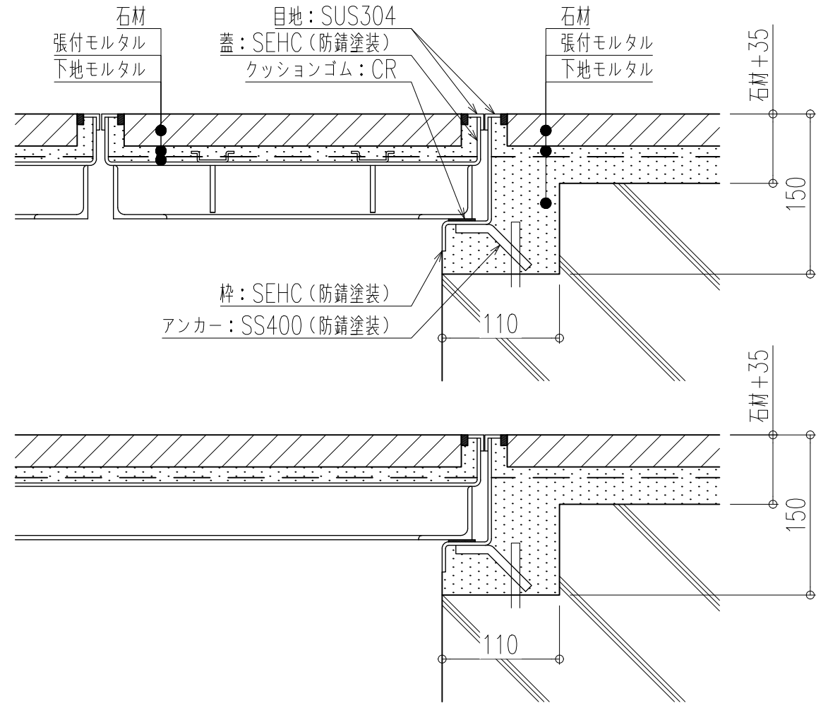
施工参考拡大図
